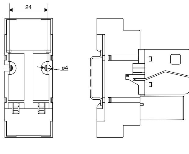
Рисунок 2. Реле модульное серии РП30 с креплением на DIN-рейку 35 мм
